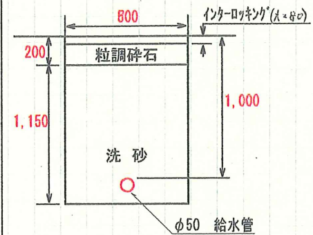
道路掘削復旧断面図
