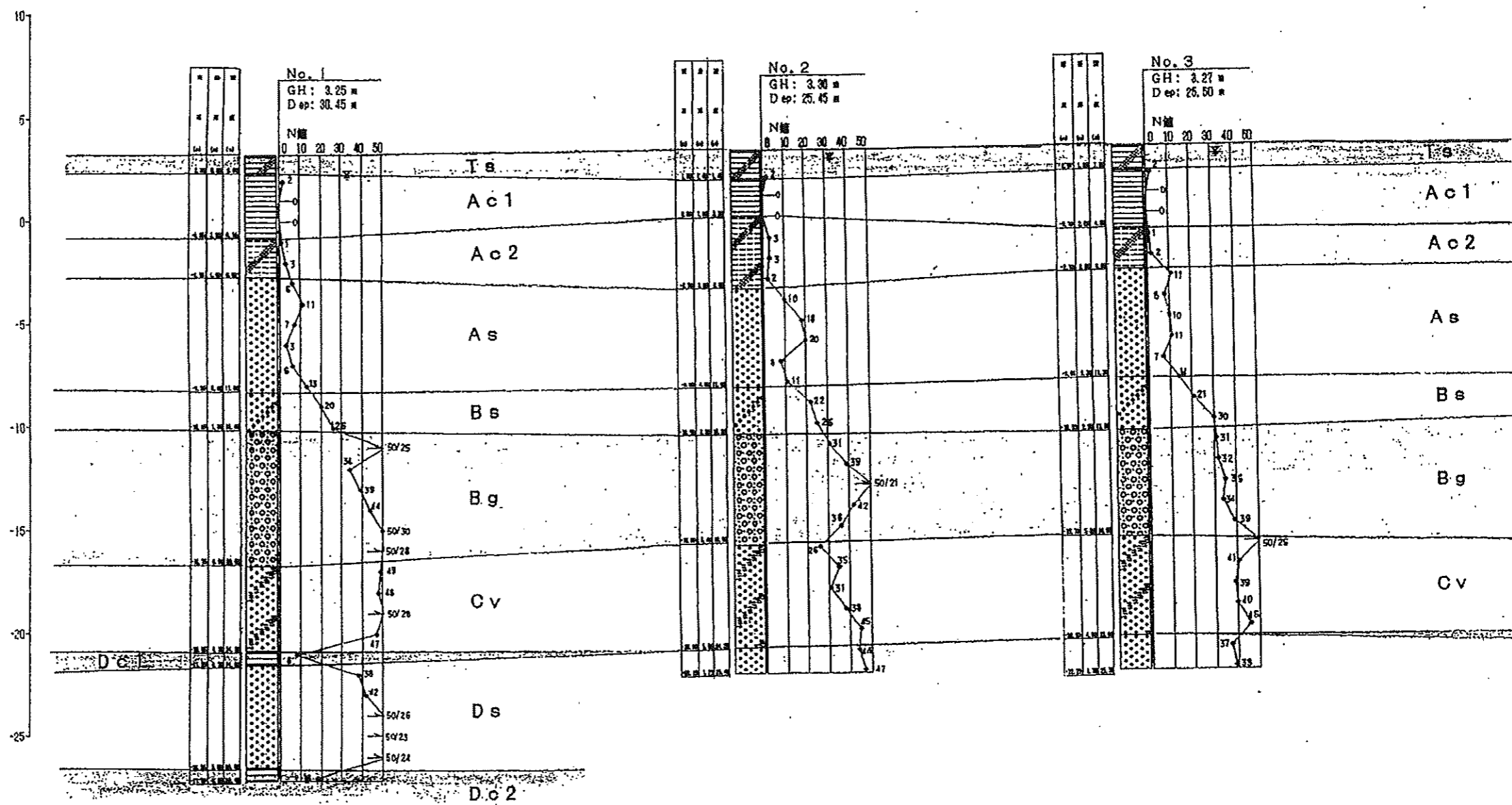
推定地質断面図
