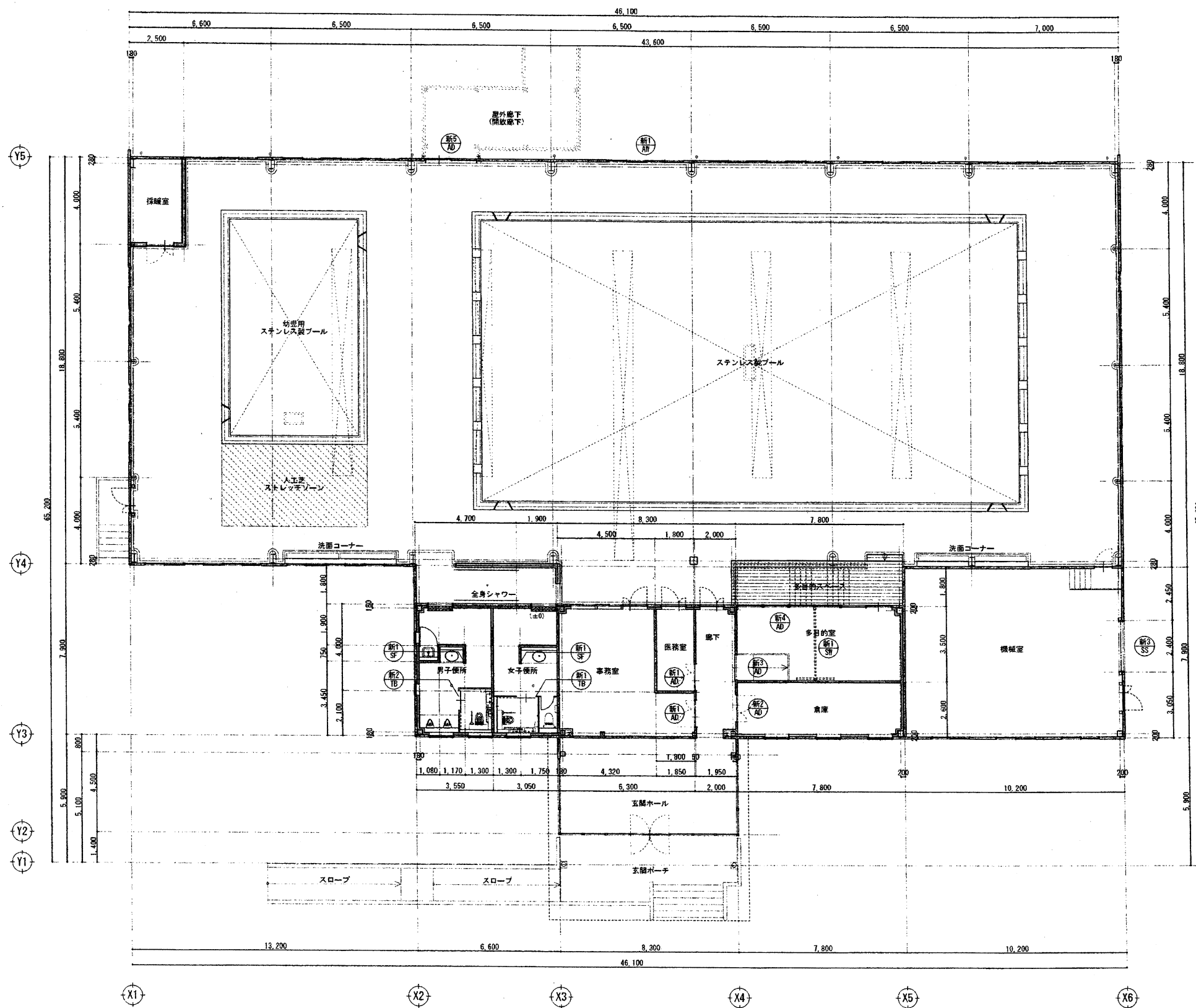
改修1階平面図 1/200 (A3)
